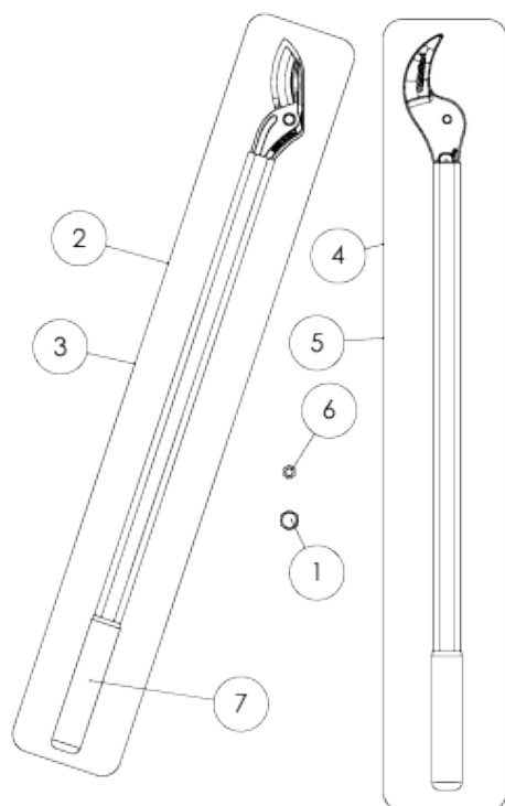
ESPLOSO TRONCARAMI 80-100_REV00
