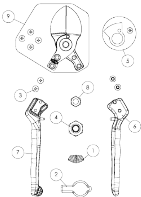
ESPLOSO B12_REV00
